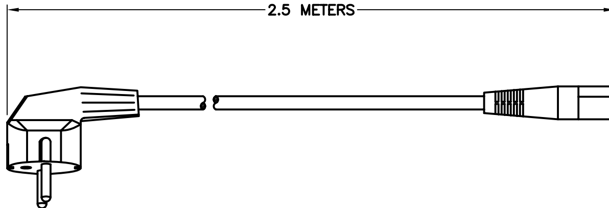
IEC 60320. C-13
